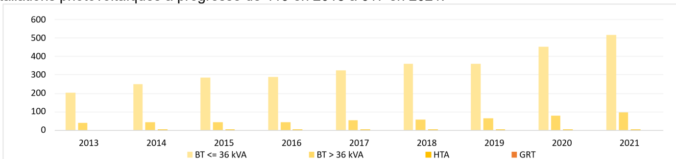
Evolution du nombre d'installations photovoltaïques par segment sur le territoire de Cauvaldor (source : ORCEO, AREC Occitanie)
