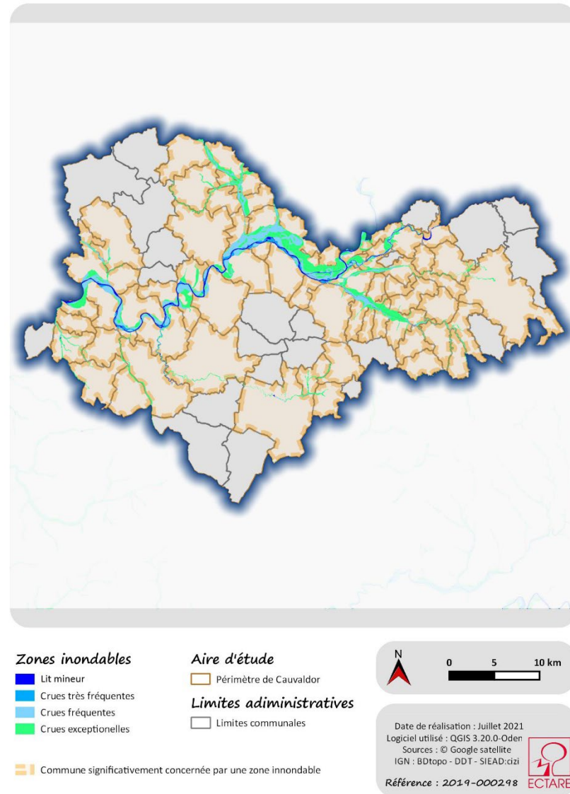
Carte 15 : Zones inondables (CIZI hors PPRI)
