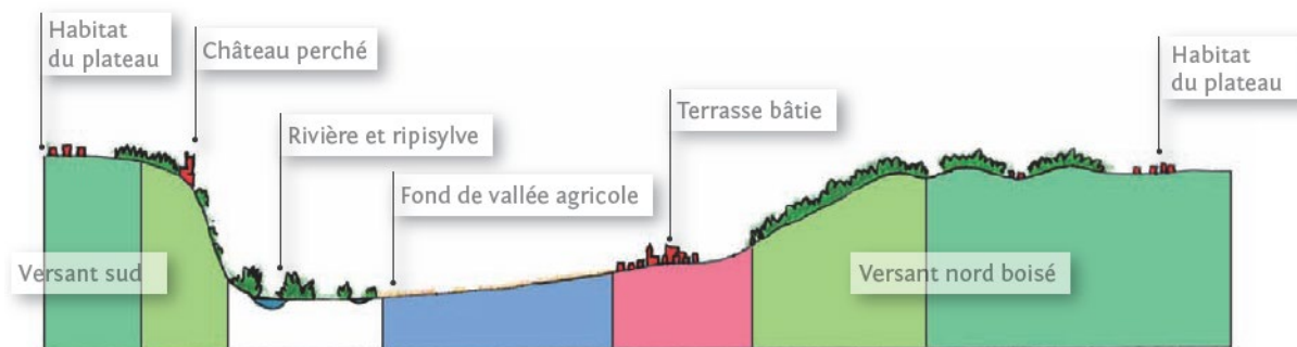
Illustration 40 : Coupe illustrant le principe théorique de l'organisation étagées d'une boucle de vallée (Source : CAUE 2010)
