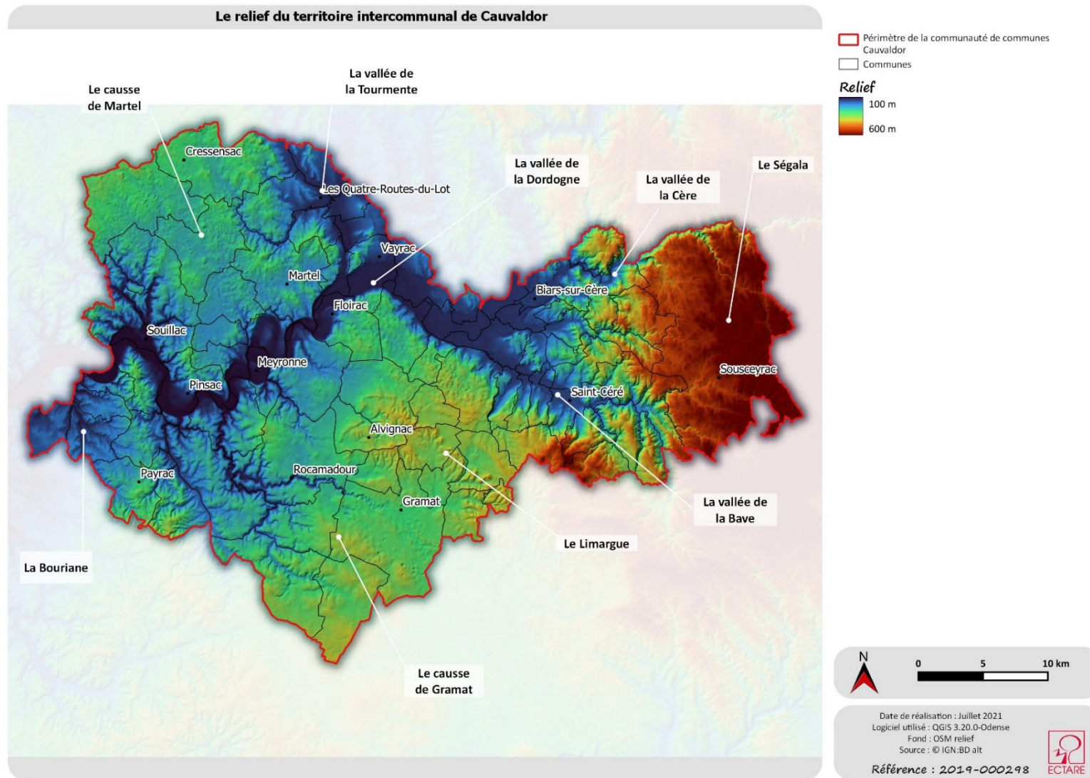
Carte 3 : Le relief du territoire
