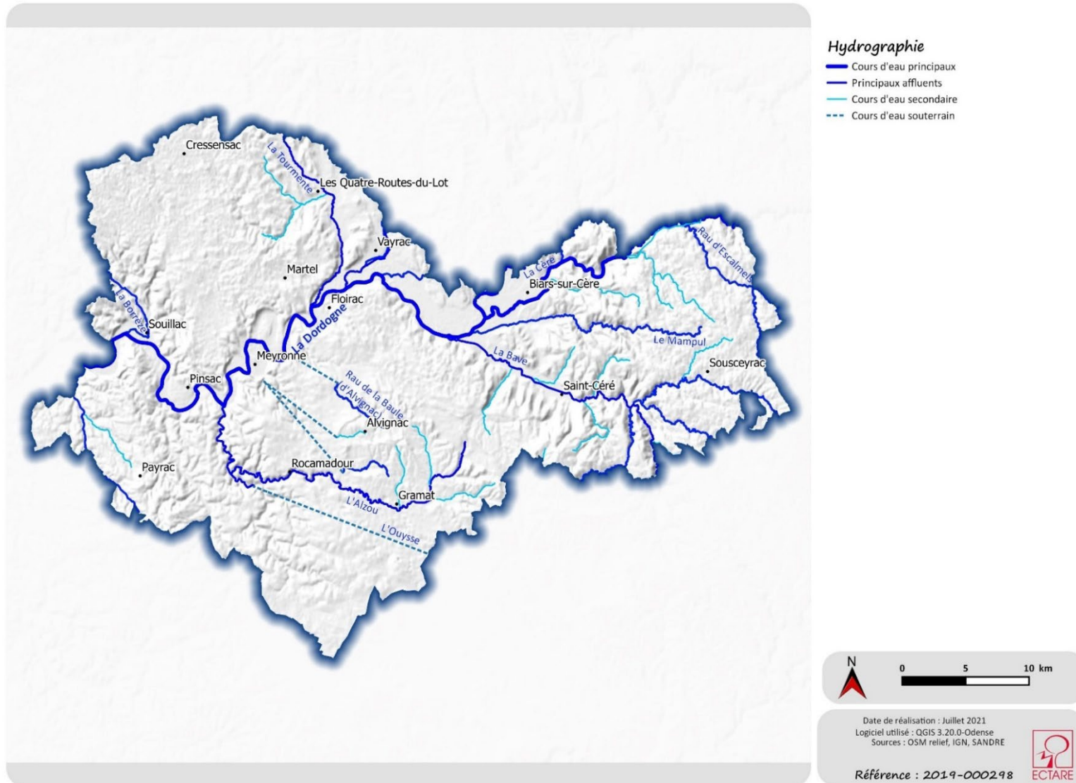
Carte 10 : Réseau hydrographique
