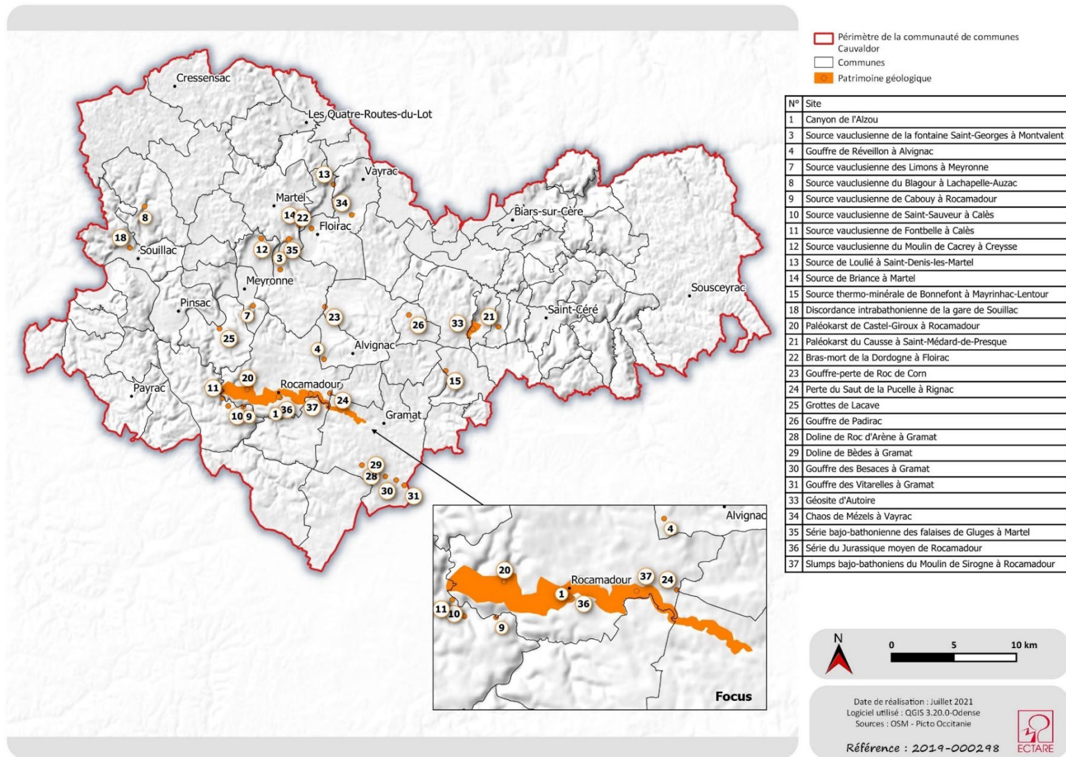
Carte 6 : Carte du patrimoine géologique
