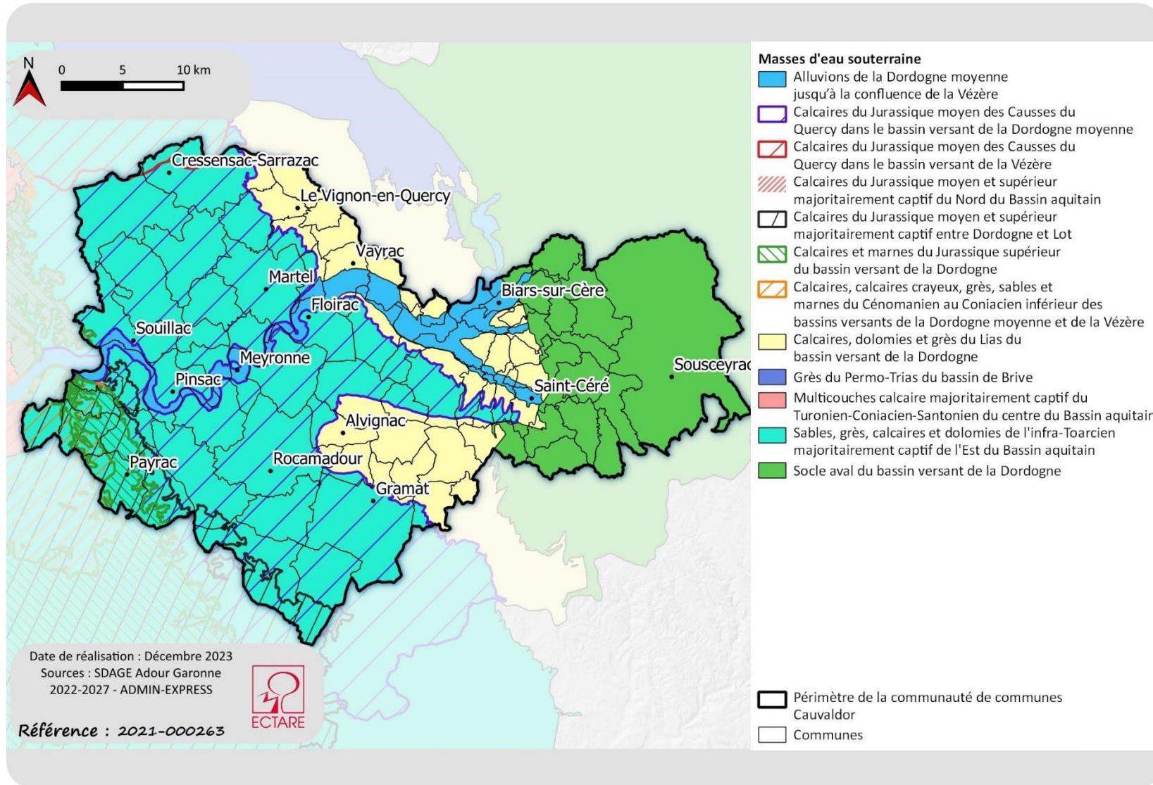
Carte 7 : Carte des masses d'eau souterraines
