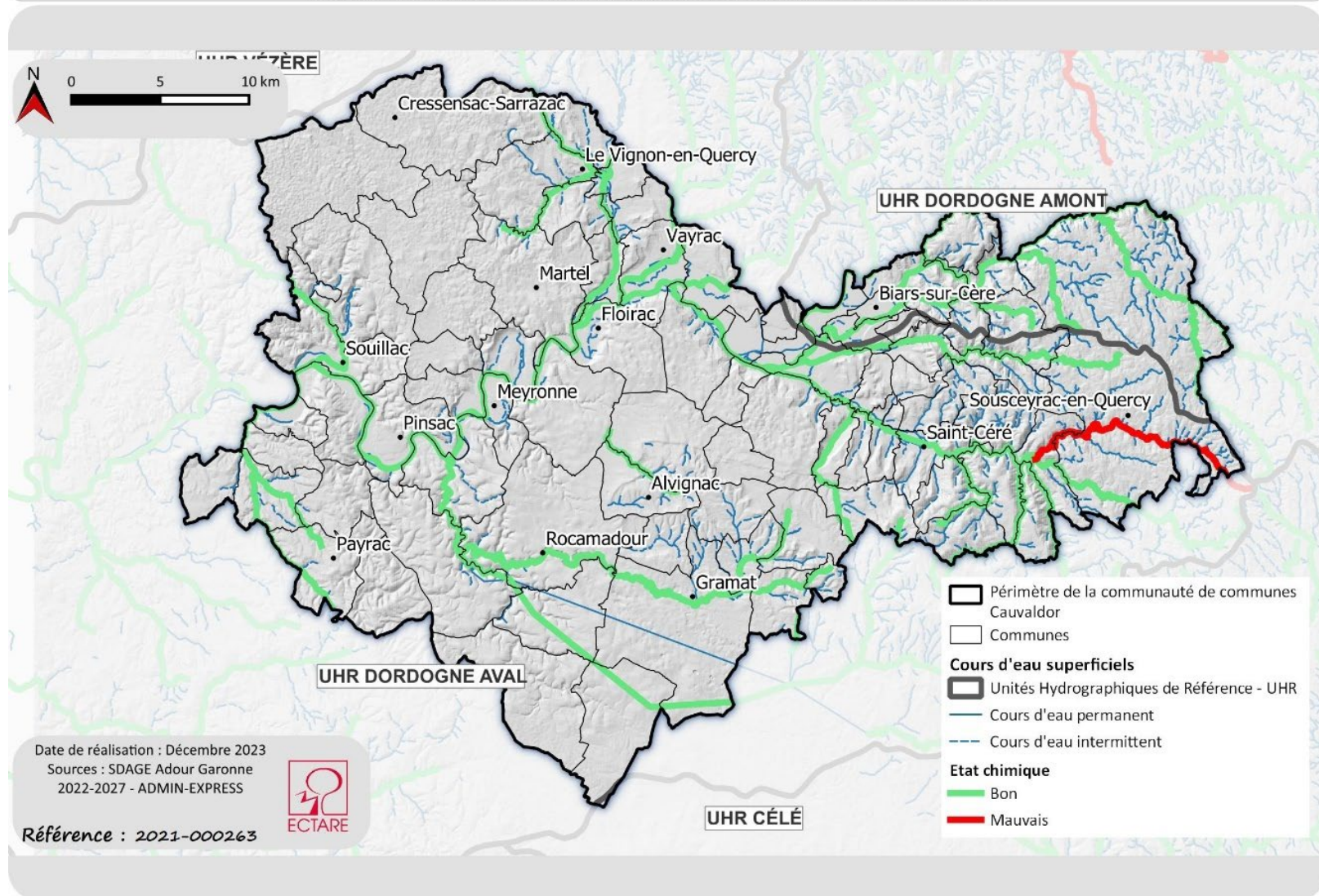
Carte 13 : Etat chimique des masses d'eau superficielles
