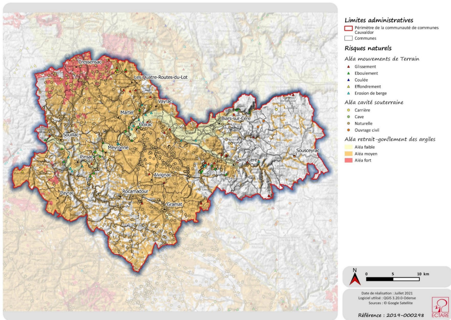
Carte 19 : Localisation des risques naturels (hors inondations)
