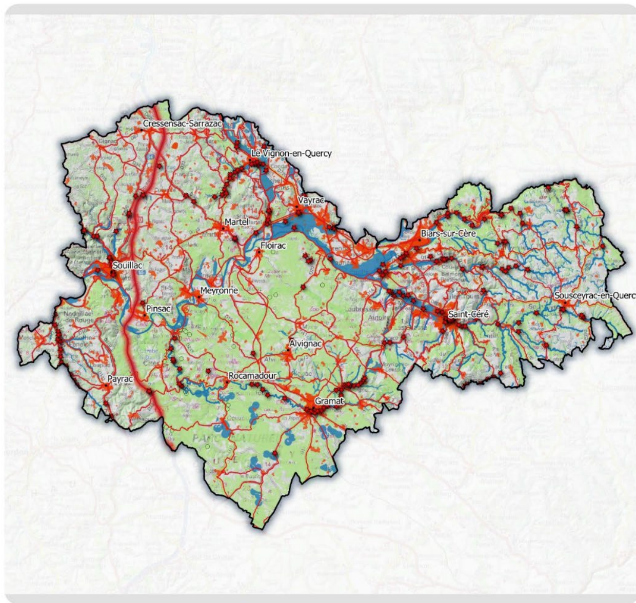
Carte 38 : Trame Verte et Bleue du PLUi-H
