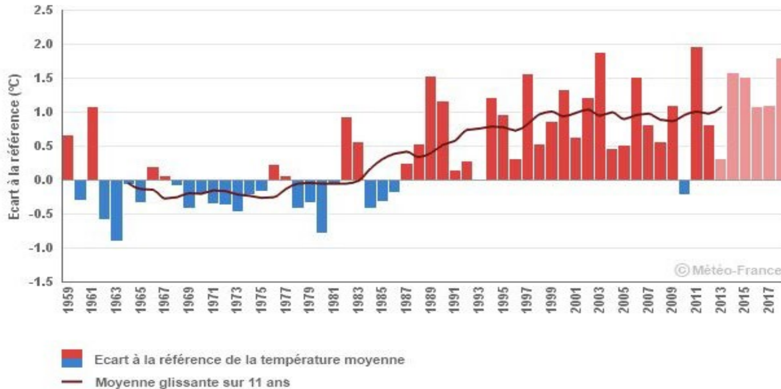
Illustration 5 : Température moyenne annuelle : écart à la référence 1961-1990 à la station de Gourdon (Source : Météo France – Climat HD)
